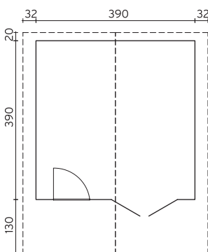
Bordeaux 1 Art.-Nr.: FRF40-4141
