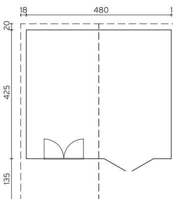
Bordeaux 2 Art.-Nr.: FRI40-5044
