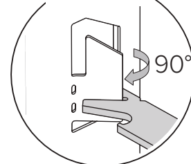
H Paroi / Wand / Wall / Wand
