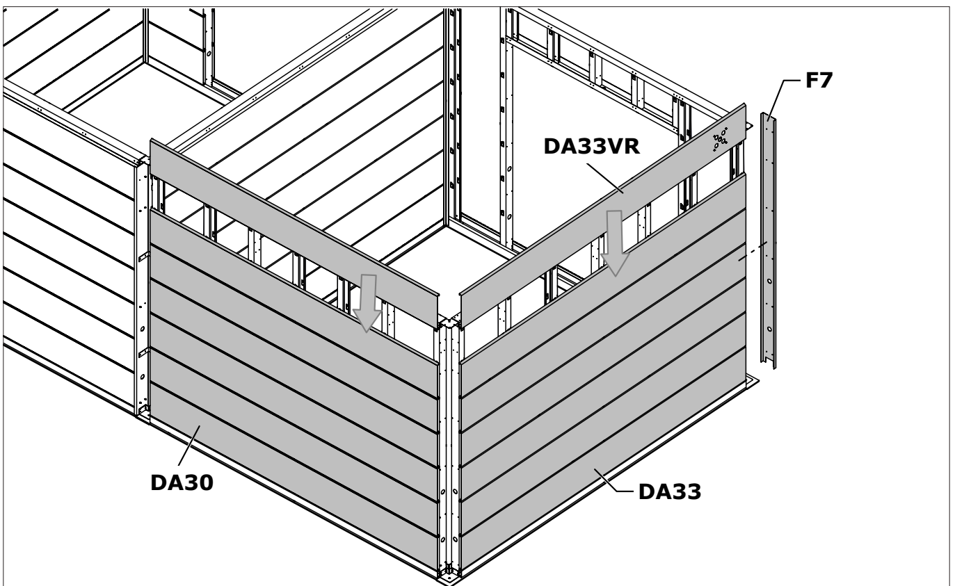
B1/B2/CD1/D2 Paroi / Wand / Wall / Wand
