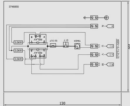
Commande interne du poêle pour sauna 9 kW
