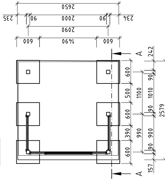
Grundriss
