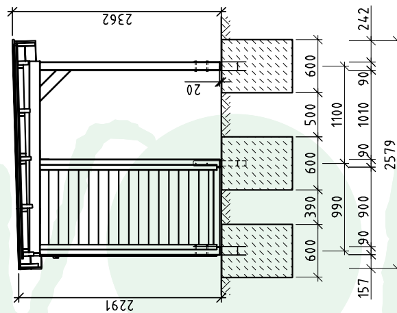
Schnitt A-A
