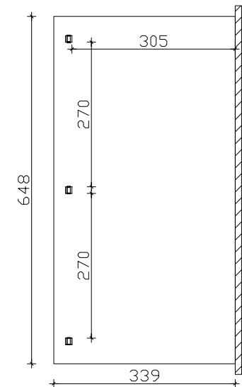
Grundriss
