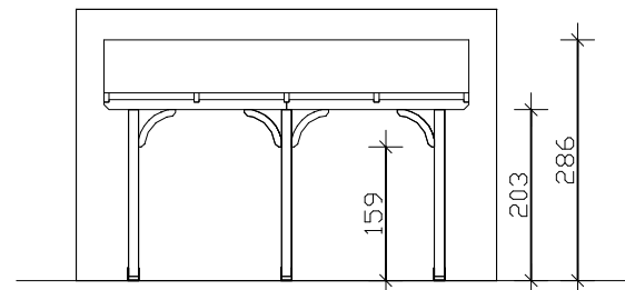
Fronansicht
