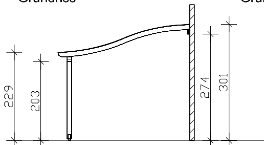
Seitenansicht
